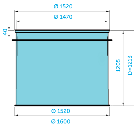
TECHNOLOGICKÁ ŠACHTA PRO INSTALACI FILTRACE A PROTIPROUDU
