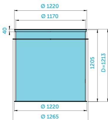
TECHNOLOGICKÁ ŠACHTA PRO INSTALACI FILTRACE
