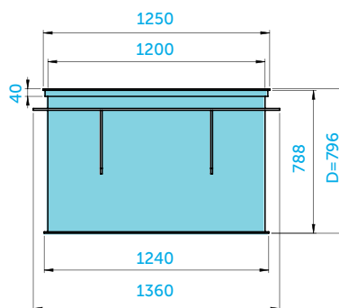
TECHNOLOGICKÁ ŠACHTA PRO INSTALACI PROTIPROUDU
